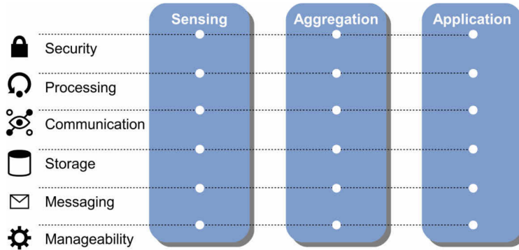
Abb. 5. Grundlegender Zusammenhang der horizontalen und vertikalen Ebenen in Sensorischen Systemen
