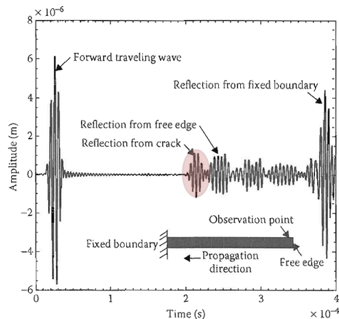
Abb. 4. Zeitaufgelöste Ultraschallsignale (geführte Wellen) in der Schadensdiagnostik
