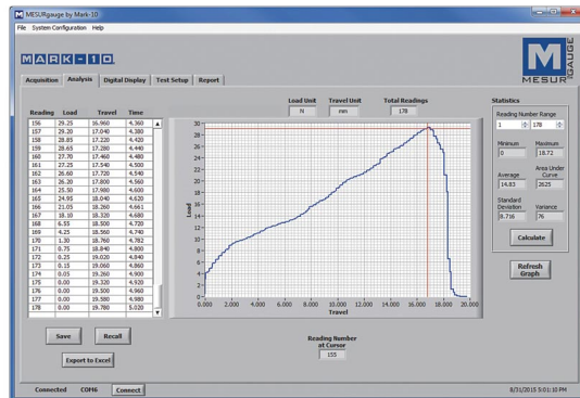
Abb. 3. Dehnungsversuch mit Dehnungs-Kraft Diagramm
